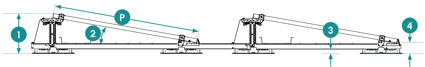
Zij aanzicht
