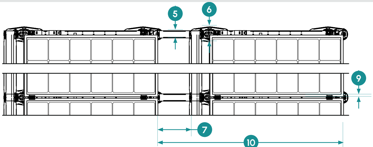
Boven aanzicht
